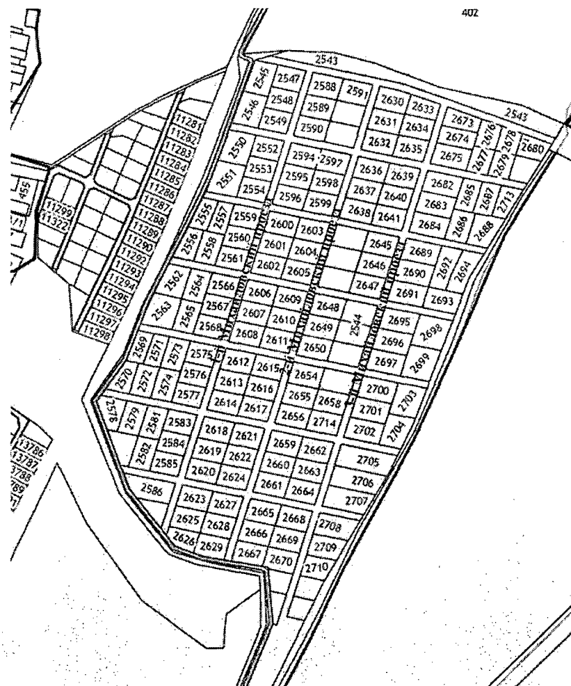
Схема элементов улично-дорожной сети в деревне Малевка муниципального образования городской округ город Тула
